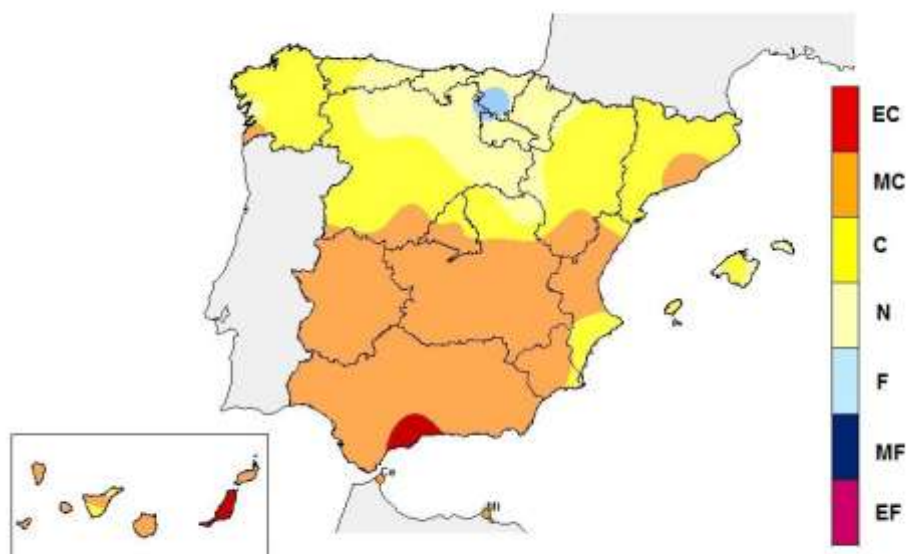
CARACTER DE LA TEMPERATURA - MAYO 2014
