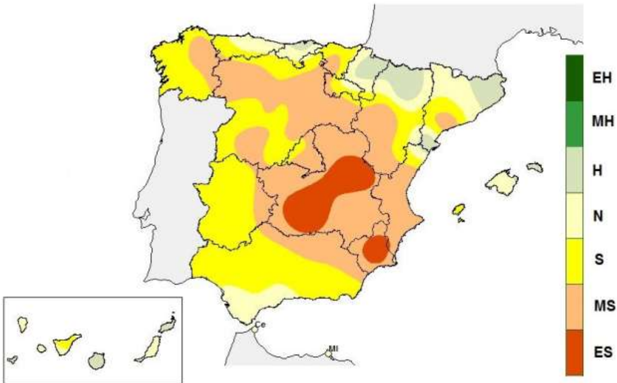
CARACTER DE LA PRECIPITACIÓN - MAYO 2014
