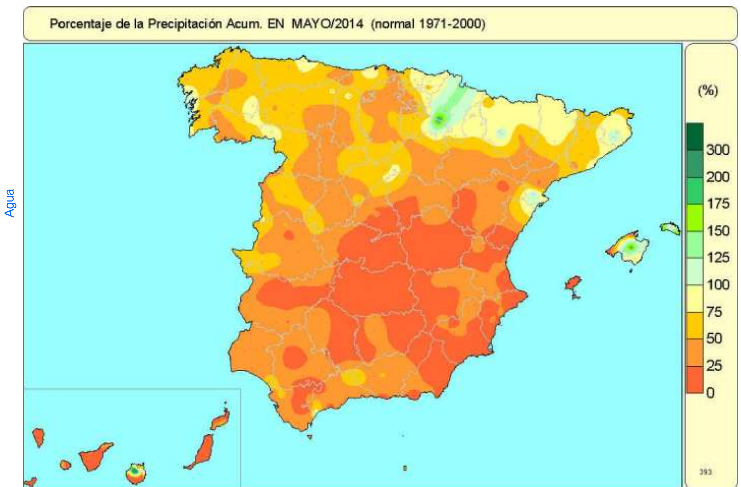
Porcentaje sobre el valor medio normal (1971-2000) de la precipitación acumulada en el mes de mayo de 2014.
